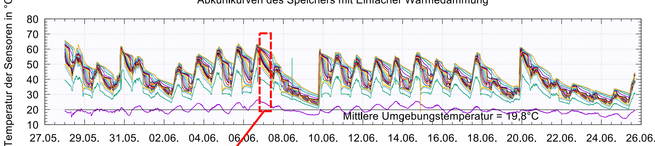
Abkühlkurven des Speichers mit Einfacher Wärmedämmung
