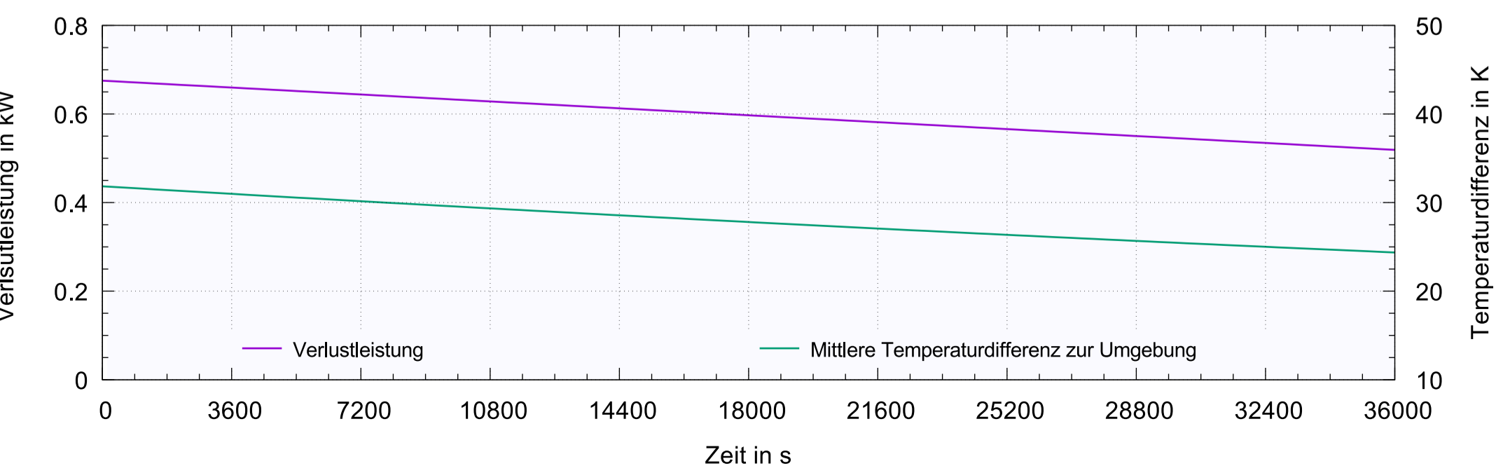
Verlustleistung des Wärmespeichers und mittlere Temperaturdifferenz zur Umgebung
