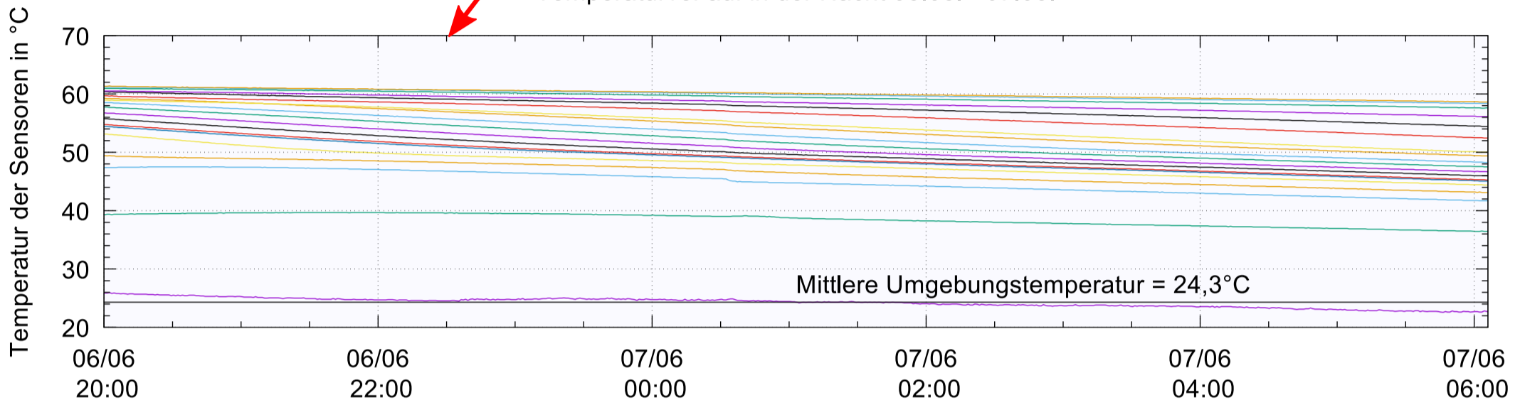
Temperaturverlauf in der Nacht 06.06. - 07.06.
