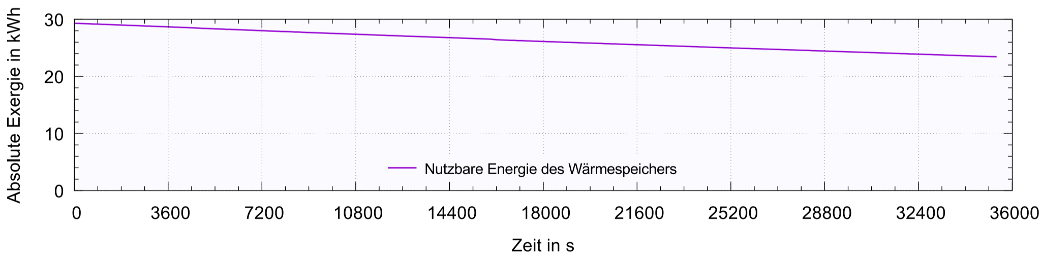
Exergiegehalt (zu 20°C) des Wärmespeichers über die Nacht
